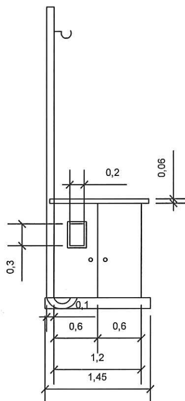
ΕΜΠΡΟΣΘΙΑ ΟΨΗ
